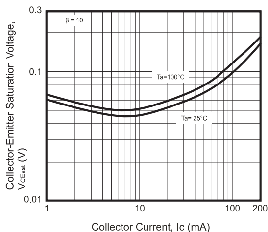
Fig.4 - V_{CEsat} — I_C
